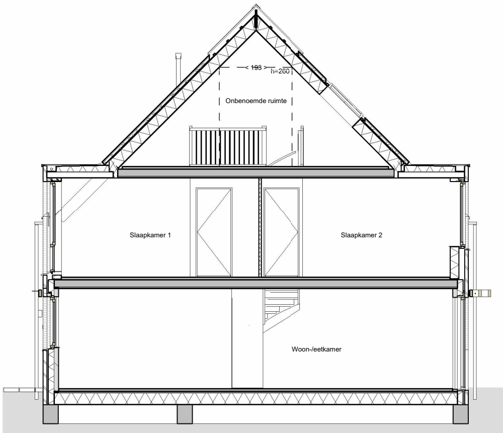
doorsnede
