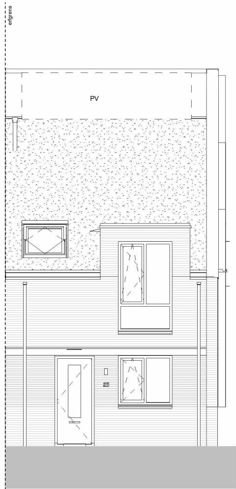
voorgevel
