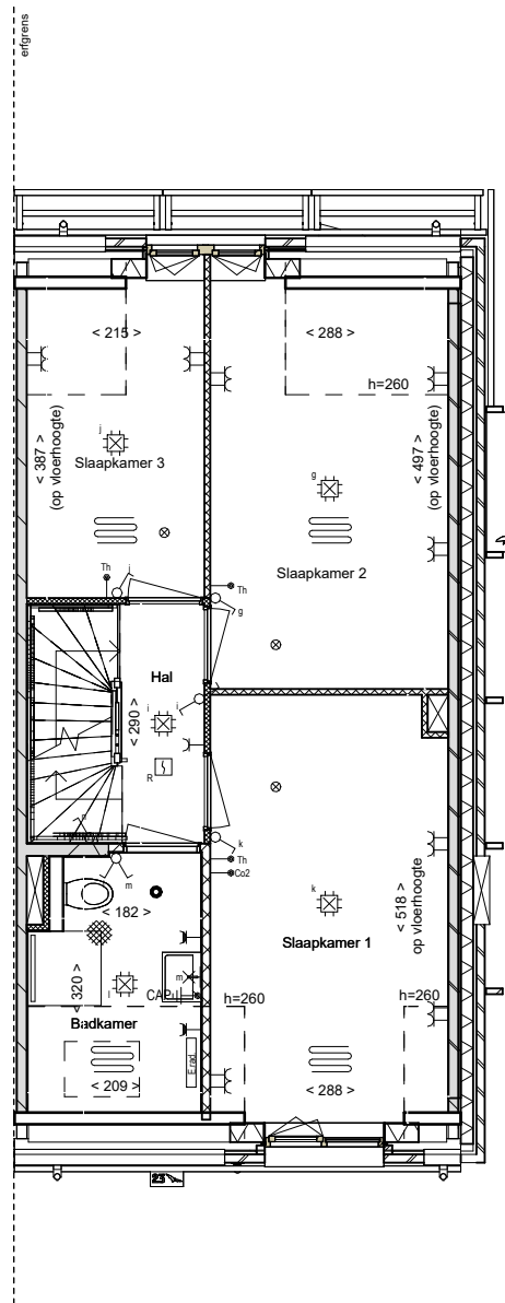
01 eerste verdieping
