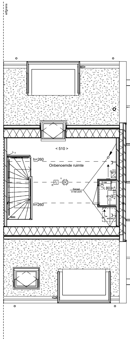
02 tweede verdieping
